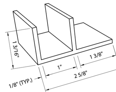
F-BRACKET DETAIL SCALE: N.T.S.
